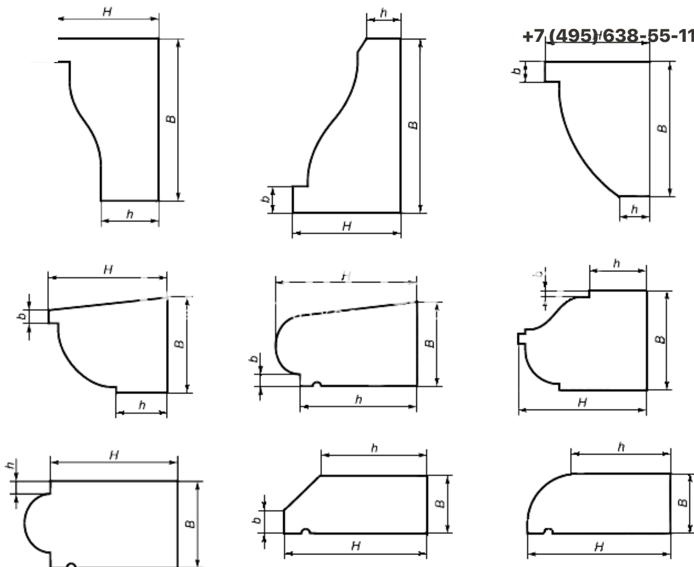
Профили кордонных камней по ГОСТ 23342-2012 (рис. 4)
